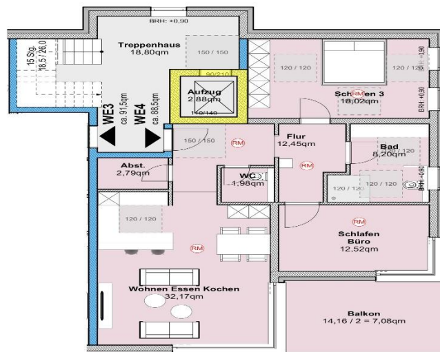
Grundriss 1. OG WE 4
