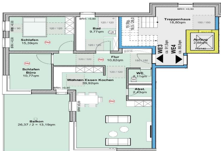
Grundriss 1. OG WE 3
